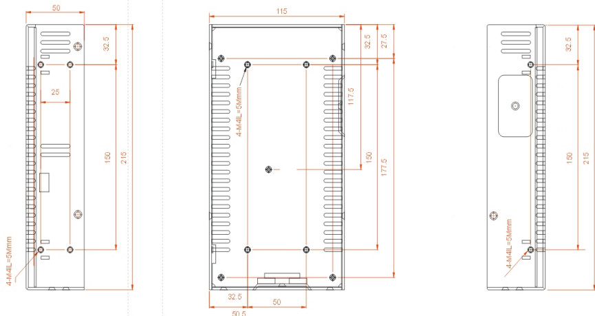
■12#机构尺寸(单位: mm) 215x115x50
