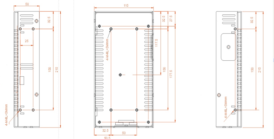
■12#机构尺寸(单位: mm) 215x115x50
